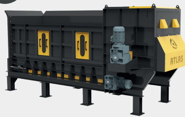
GERİ DÖNÜŞÜM PAKET AÇMA MAKİNASI RECYCLING PACKAGE OPENER MACHINE
