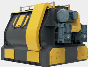
ÇİFT ŞAFTLI MİKSER DOUBLE SHAFT MIXER
